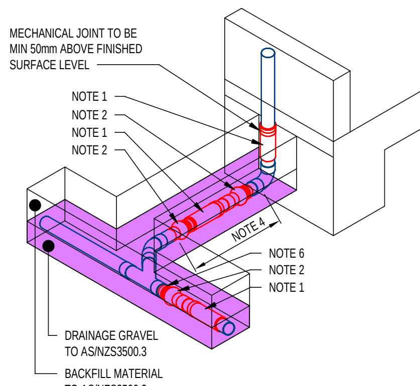
2 STORMWATER DOWNPIPES N.T.S.
